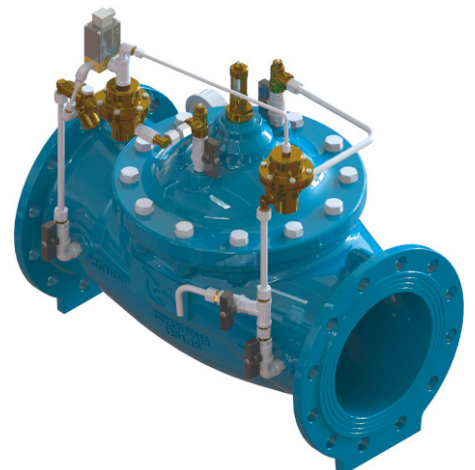
M3700 [DN300 to DN1000] ODCIĘCIE PRZEPŁYWU STEROWANE ELEKTRYCZNIE
