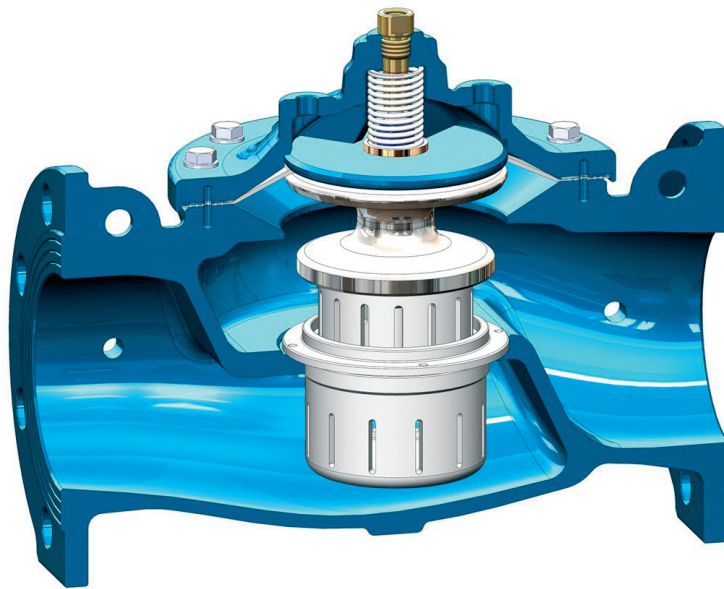
PODWÓJNY CYLINDER SZCZELINOWY
