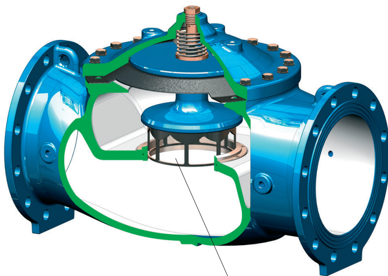
V-PORT Konfiguracja zaworu głównego
