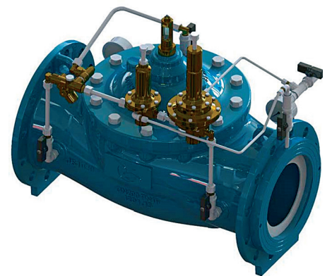
M3410 OGRANICZENIE PRZEPŁYWU WRAZ Z REDUKCJĄ CIŚNIENIA WYJŚCIOWEGO
