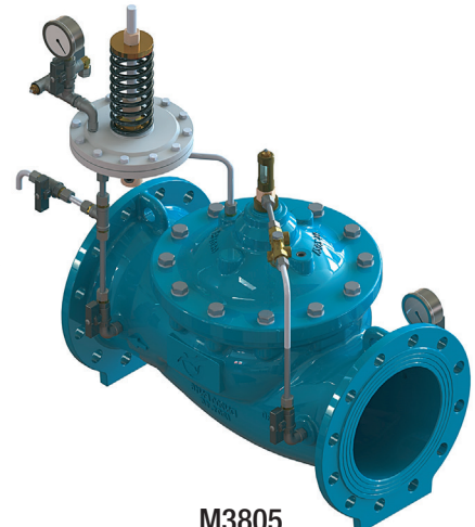
M3805 REGOLAZIONE A LIVELLO COSTANTE PIEZOMETRICA UNIDIREZIONALE
