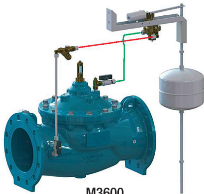
M3600 SEZIONAMENTO A GALLEGGIANTE
