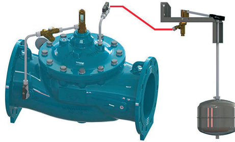
M3500 REGOLAZIONE LIVELLO COSTANTE A GALLEGGIANTE
