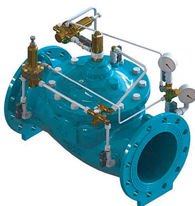
M3219 SFIORO DELLA PRESSIONE CON APERTURA ANTICIPATA
